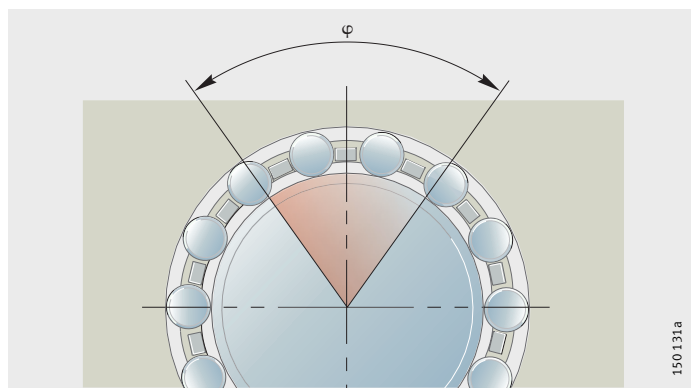
Figura 8 Angolo di oscillazione φ
