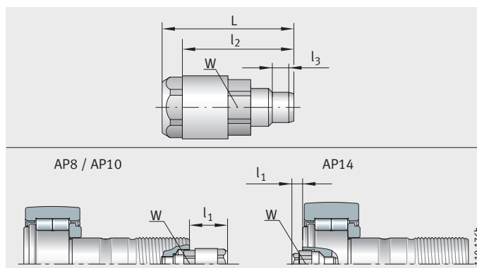
Figura 11 Adattatore di lubrificazione centralizzata - Dimensioni
