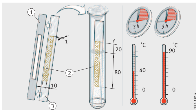
Figura 7 Idrorepellenza secondo norma DIN 51 807
