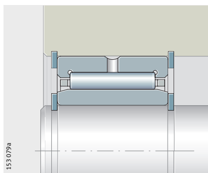
NKI Figura 1 Fissaggio assiale tramite anelli elastici
