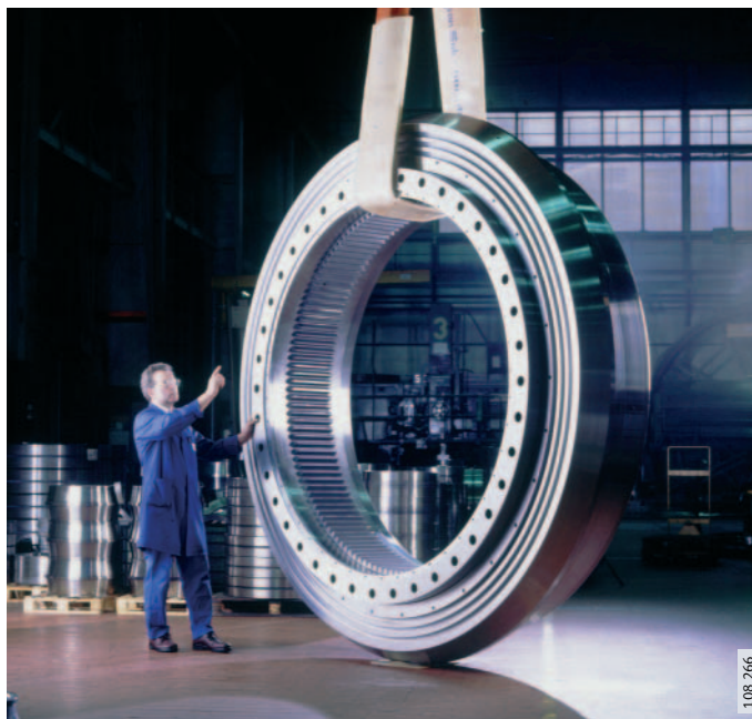
Figura 12 Cuscinetto combinato, radiale ed assiale a rulli cilindrici con corona dentata integrata
