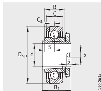
GSH..-2RSR-B
