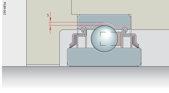
Figura 3 Gioco d'esercizio
