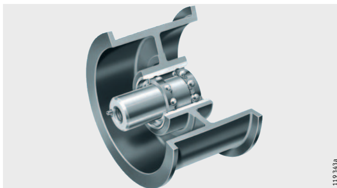
Figura 3 Rullo tendicinghia a rumorosità ottimizzata per ritorcitori
