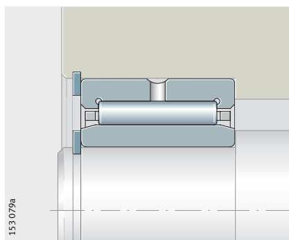
NKI Figura 2 Fissaggio assiale tramite anelli elastici e spallamenti
