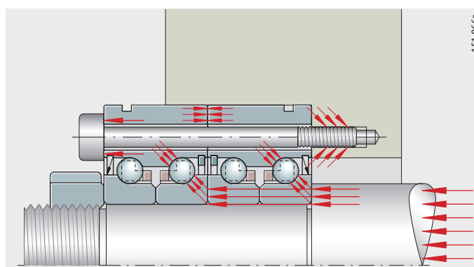
Figura 24 Carico statico assiale in direzione dell'avvitamento
