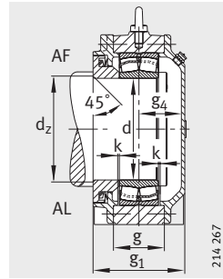
Esecuzione A Supporti con tenuta in taconite per cuscinetti con foro cilindrico
