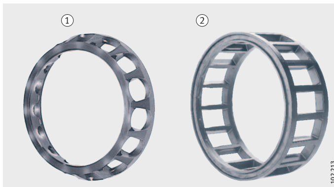
Figura 6 Gabbie massicce in poliammide rinforzata con fibre di vetro
