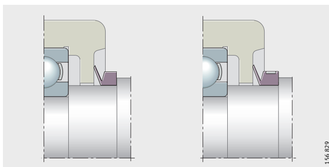
Figura 41 Anello V
