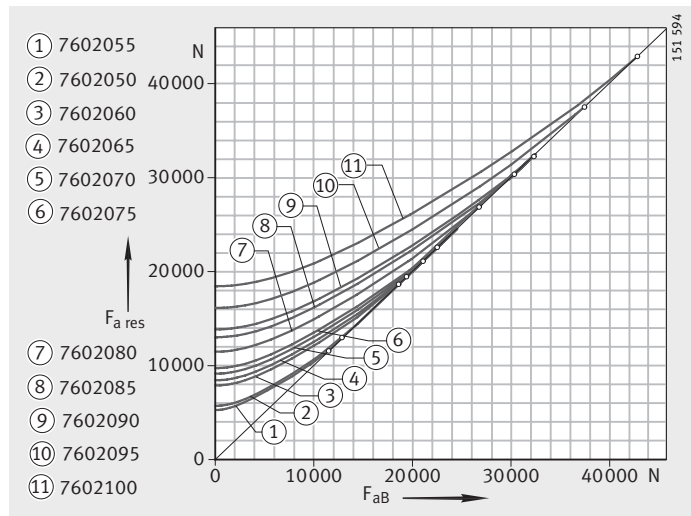
Figura 18 Carico risultante sul cuscinetto 7602050 fino a 7602100
