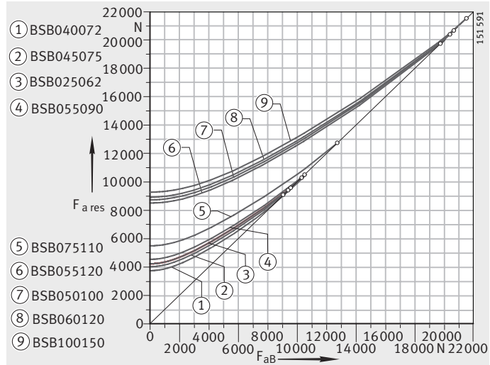
Figura 16 Carico risultante sul cuscinetto BSB
